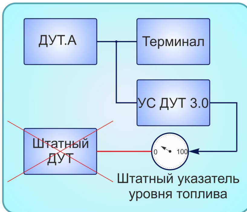
Рисунок 4 – Подключение устройства согласования УС ETS
