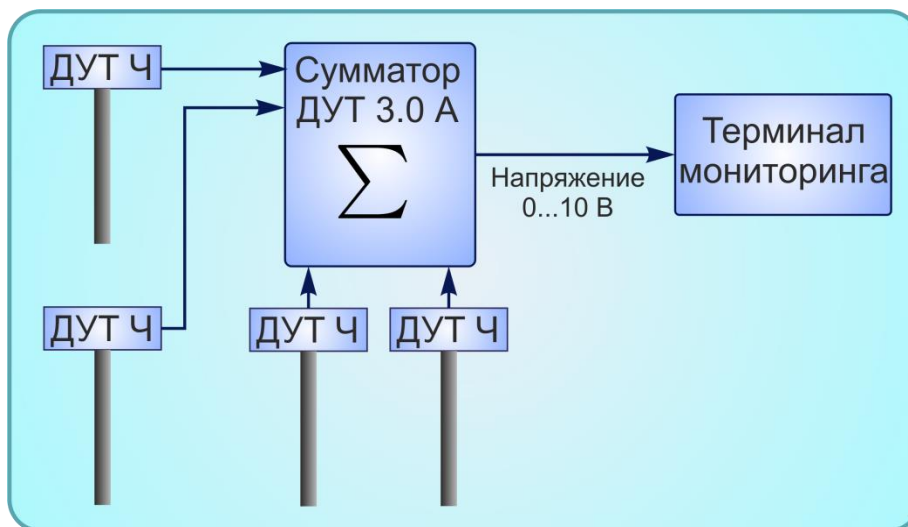
Рисунок 5 – Сумматор ETS 3.0
