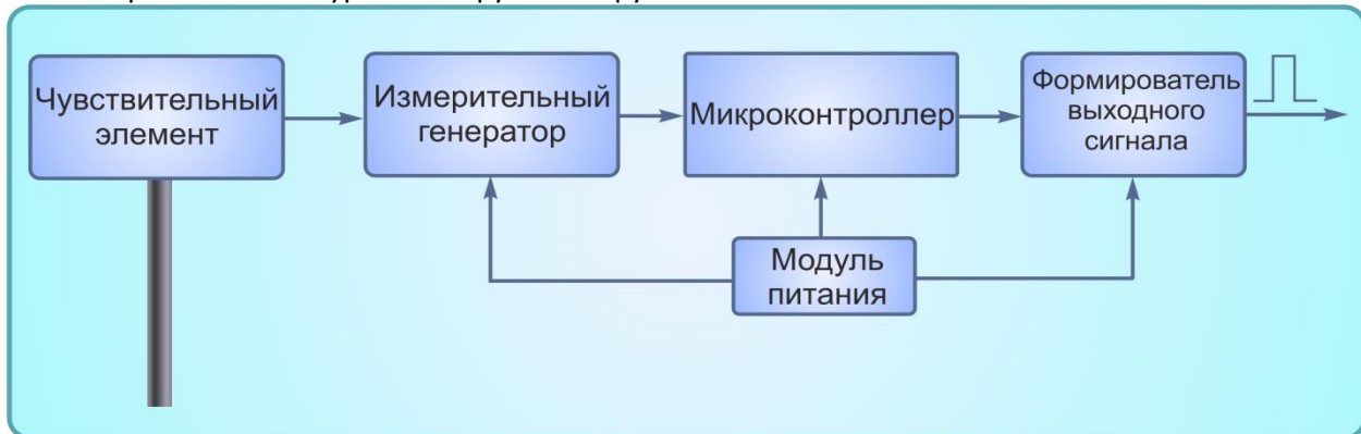
Рисунок 2 – Структурная схема ETS.A
